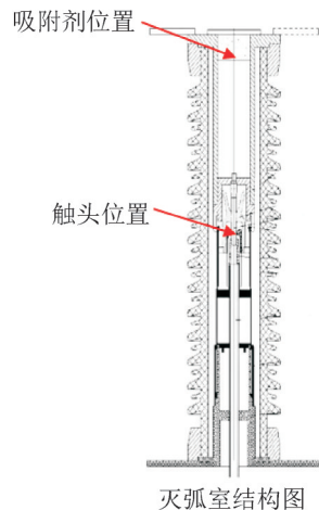
图14 灭弧室结构图 Fig. 14 Structural diagram of interrupter
