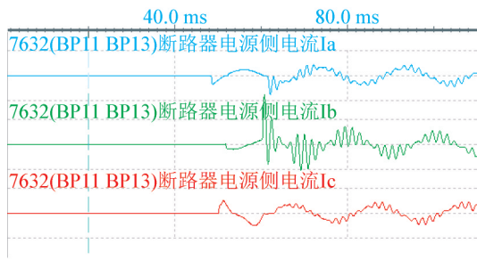
(b) 2018年2月12日 7632断路器合闸波形
