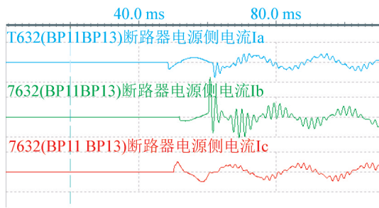
(a) 2018年2月3日 7632 断路器合闸波形
